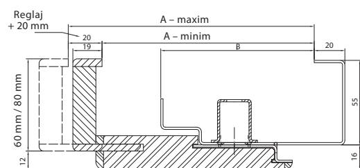
secțiune toc PROIECT Premium
