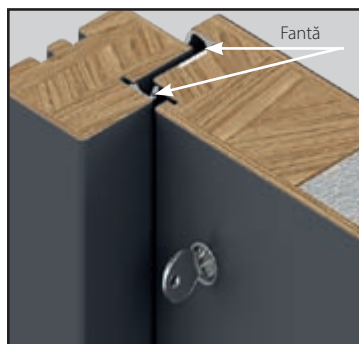
ÎNAINTE de închidere ~ 5 mm
