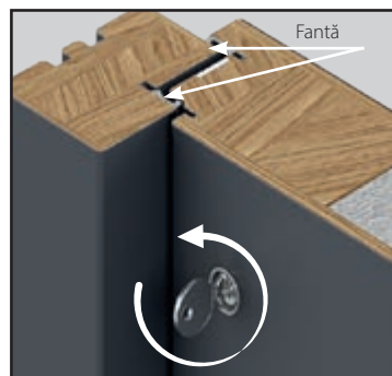
DUPĂ închidere ~ 3 mm
